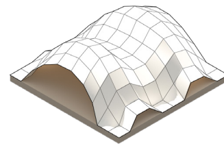
ITERATION 5 VALUE : 10.035
