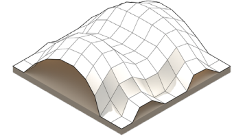
ITERATION 4 VALUE : 7.535
