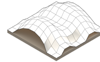
ITERATION 3 VALUE : 5.035
