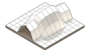
ITERATION 12 VALUE : 50.035
