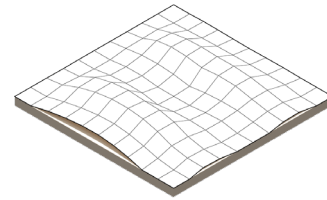
ITERATION 1 VALUE : 0.035
