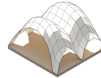
ITERATION 7 VALUE : 15.035
