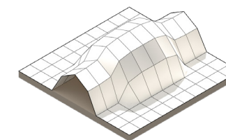
ITERATION 11 VALUE : 40.035
