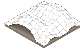
ITERATION 2 VALUE : 2.535
