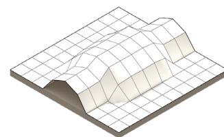
ITERATION 9 VALUE : 20.035
