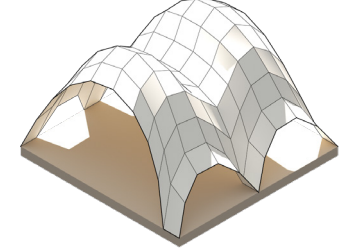
ITERATION 8 VALUE : 17.535
