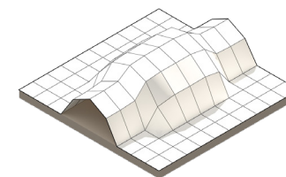
ITERATION 10 VALUE : 30.035
