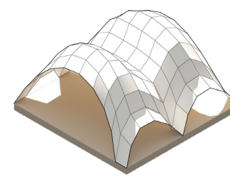
ITERATION 6 VALUE : 12.535
